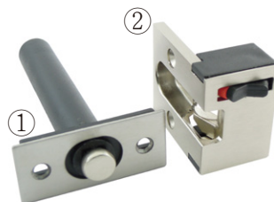
DS-1010 Zinc Alloy ①L:51 W:26 H:100 ②L:42 W:30 H:49
